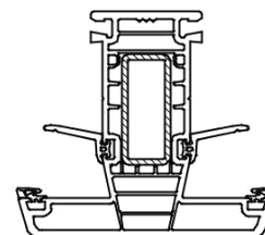
6050 tussenstijl
