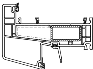
6802 bovendorpel
