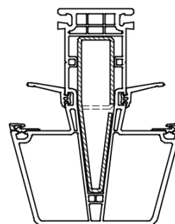
6816 tussenstijl
