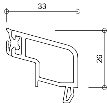
6130 glasdikte 29+30mm
