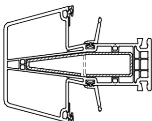
6816 tussendorpel
