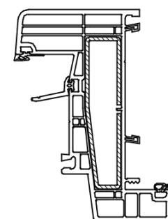
6808 buitendraaiend
