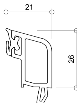
6142 glasdikte 41+42mm
