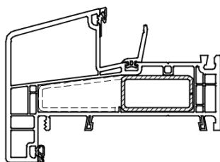
6802 onderdorpel
