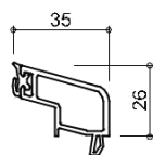
6128 glasdikte 28+29mm
