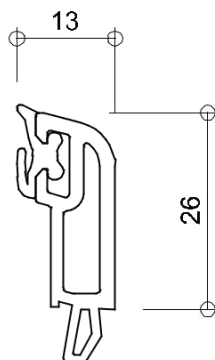
6150 glasdikte 49+50mm
