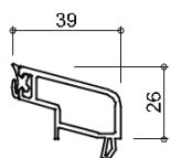
6124 glasdikte 24+25mm
