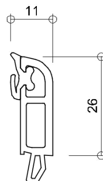
6152 glasdikte 51+52mm
