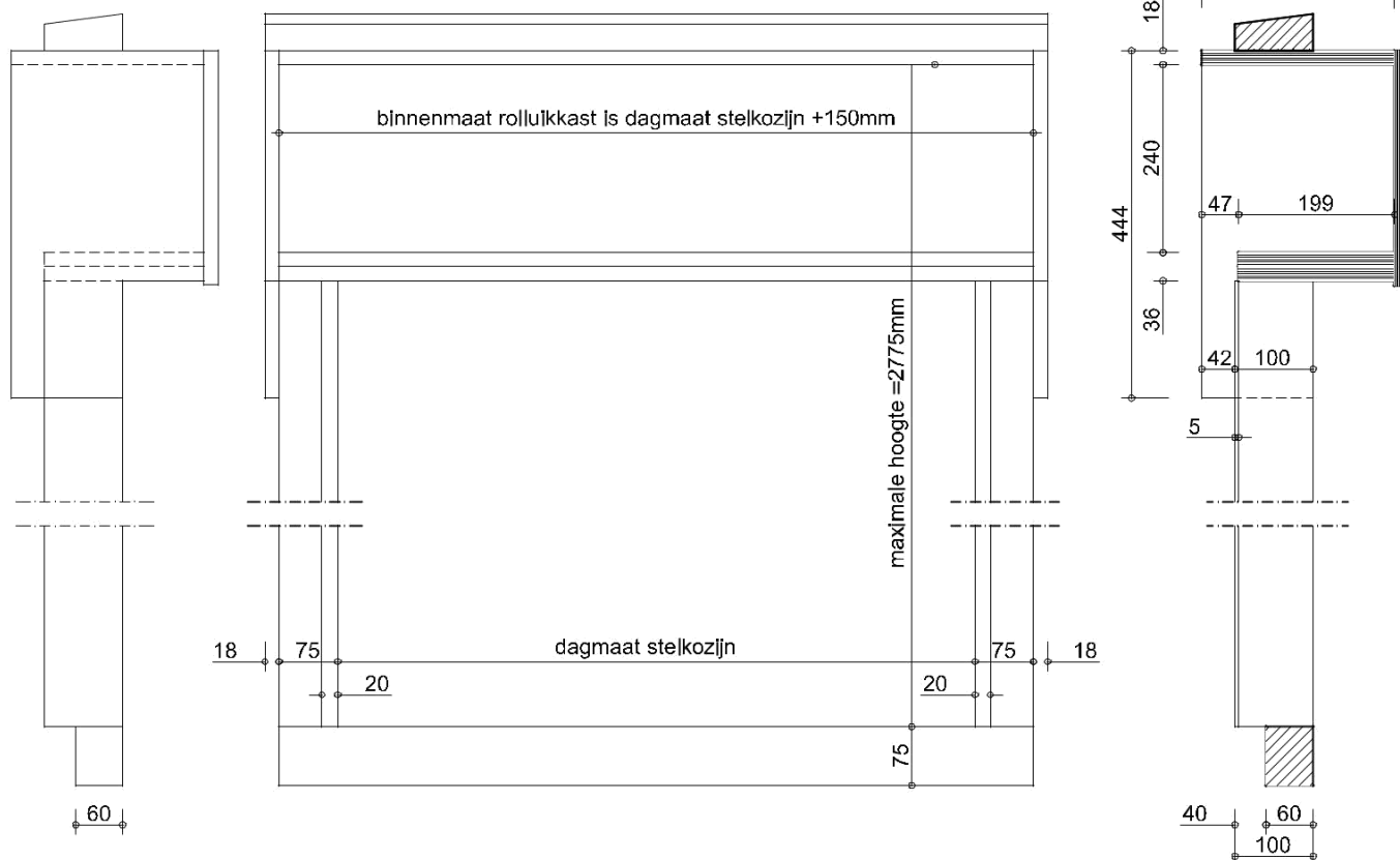
zijaanzicht
