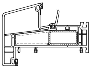
6802 onderdorpel
