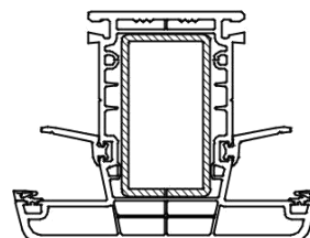
6054 tussenstijl
