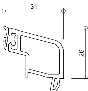
6132 glasdikte 31+32mm
