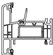
6070 onderdorpel
