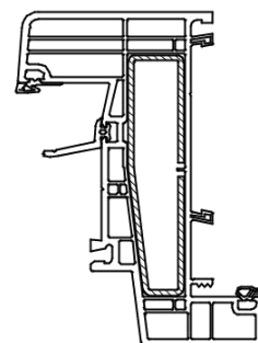
6808 buitendraaiend
