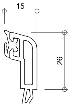
6148 glasdikte 47+48mm
