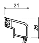
6132 glasdikte 32+33mm
