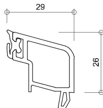
6134 glasdikte 33+34mm
